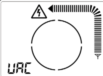
(3) Modo de identificación de la tensión de red
