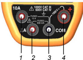
Figura 4: los terminales
