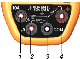
Abbildung 4: die Buchsen
