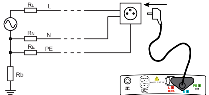
Cas d'une installation TN
