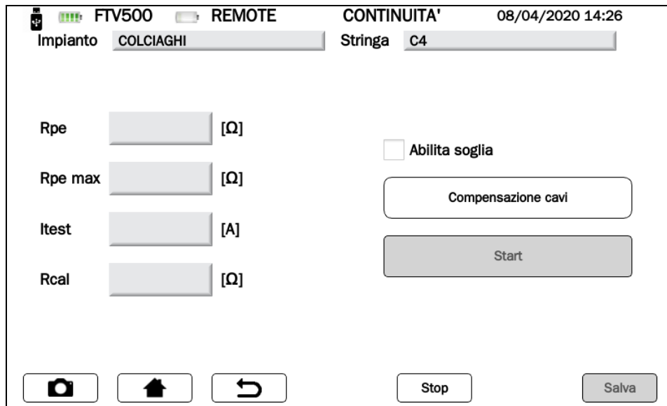
Figura 14.7.5-2 Schermata misura Continuità
