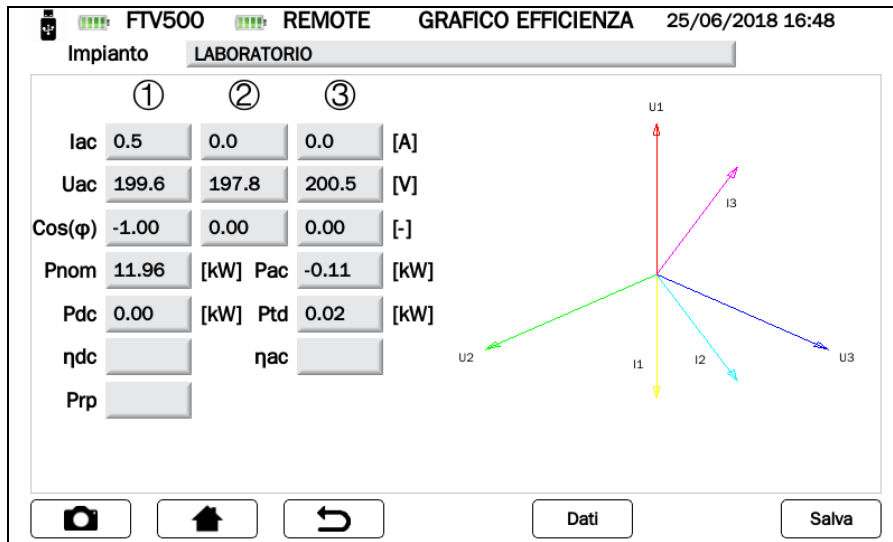
Figura 14.7.2-8 Schermata Visualizzazione Grafico Efficienza
