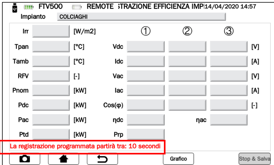
Figura 14.7.2-11 Schermata Avvio registrazione programmata in attesa
