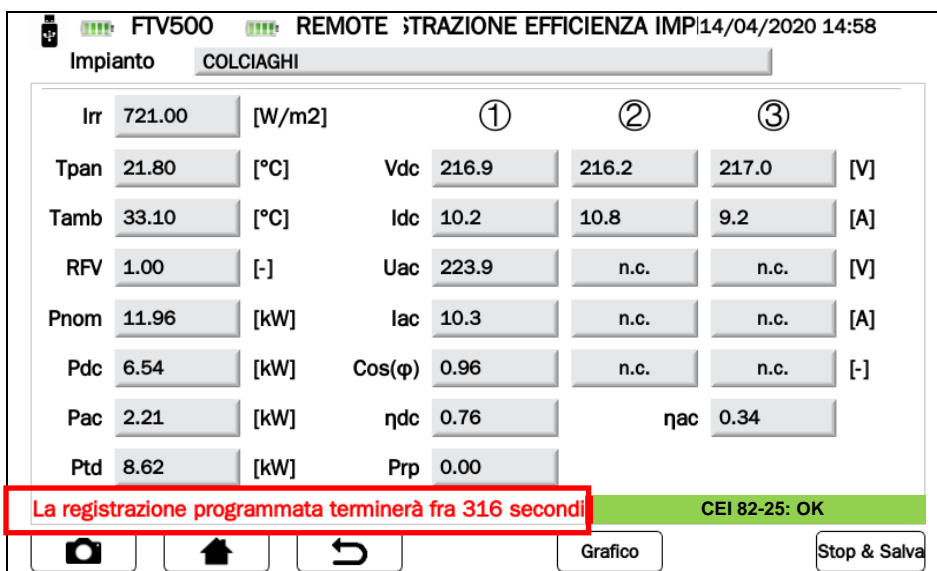
Figura 14.7.2-12 Schermata registrazione programmata in corso
