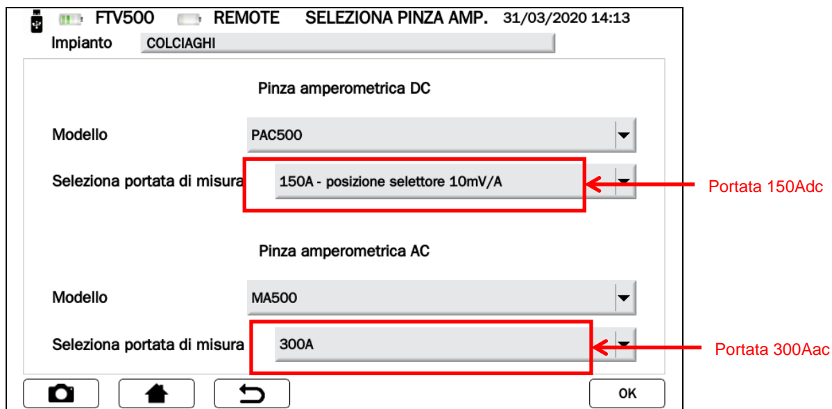
Figura 14.7.2-4 Schermata Seleziona Pinza Amperometrica
