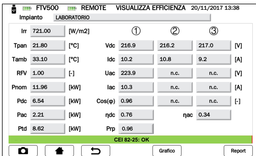
Figura 14.7.2-7 Schermata Registrazione Efficienza
