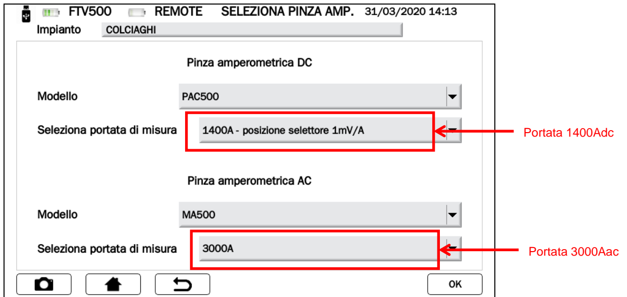
Figura 14.7.1-7 Schermata Selezione Pinza Amperometrica
