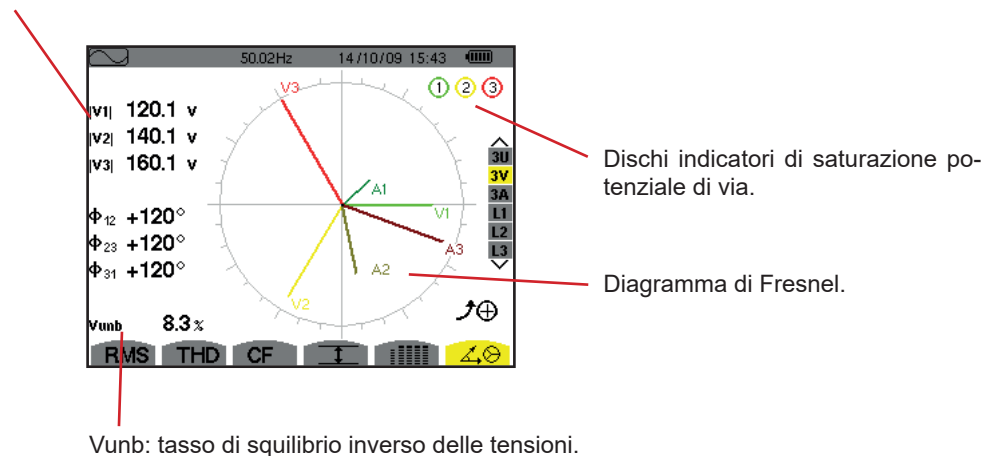
Figura 82: lo schermo di visualizzazione del diagramma di Fresnel in 3V
