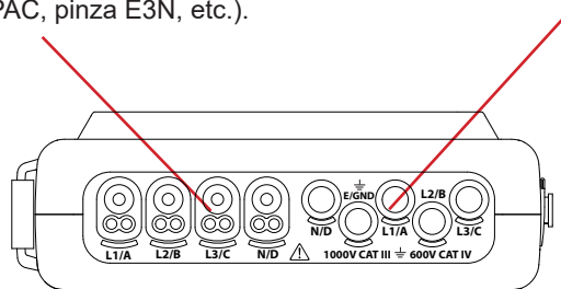
Figura 3: i morsetti di collegamento
