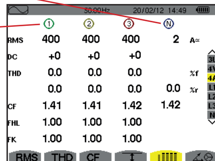
Figura 80: Lo schermo di visualizzazione simultanea in 4A
