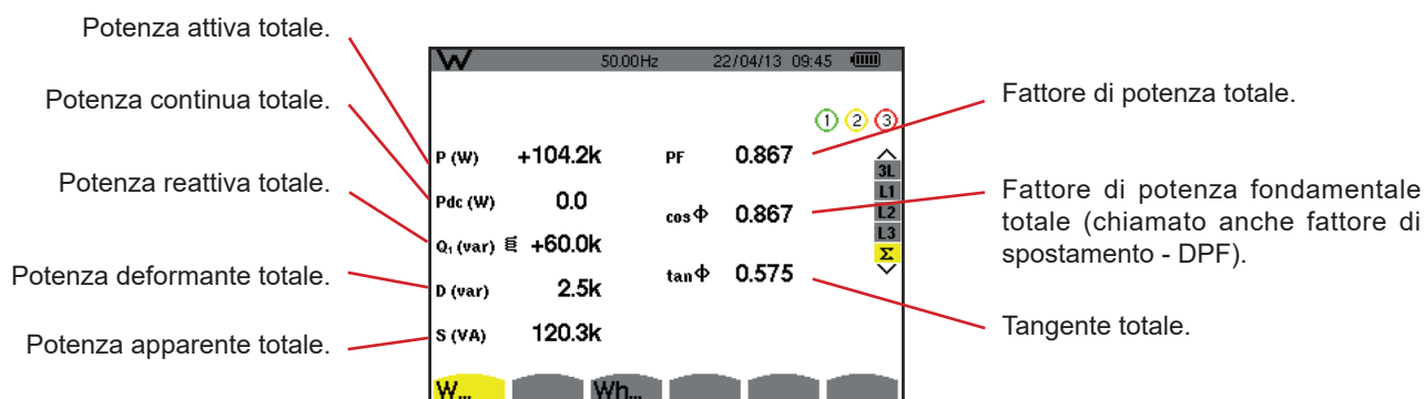
Figura 115: lo schermo di visualizzazione delle potenze e delle grandezze totali associate in \Sigma
