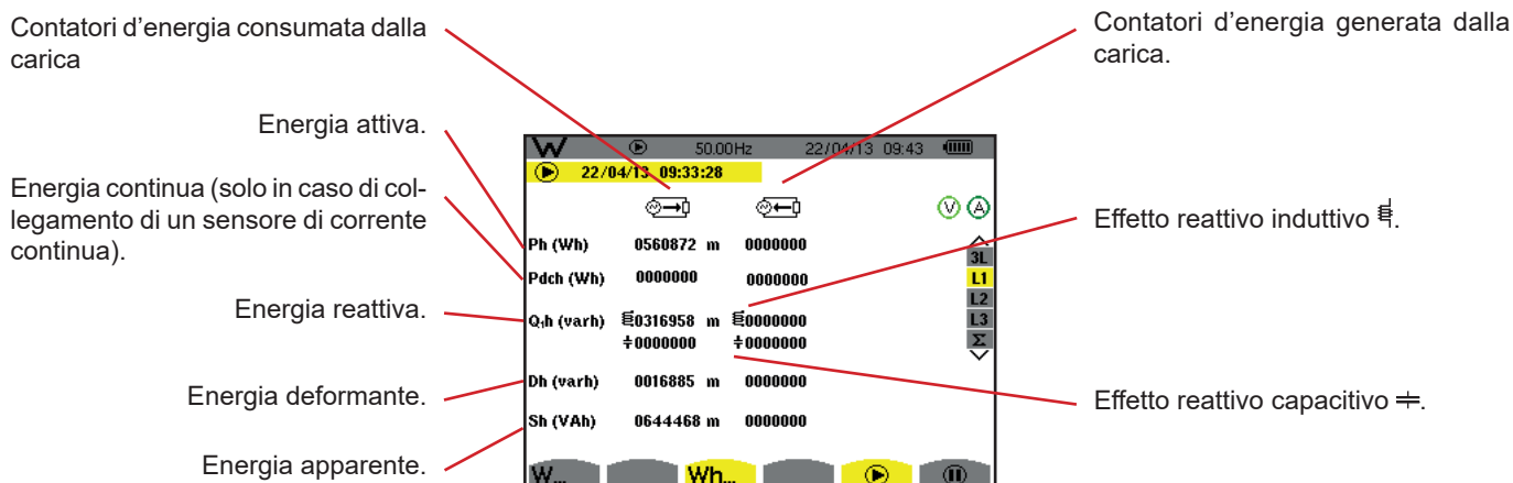
Figura 114: lo schermo di visualizzazione delle energie consumate e generate in L1
