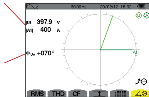
Figura 84: lo schermo di visualizzazione del diagramma di Fresnel in bifase a 2 fili
