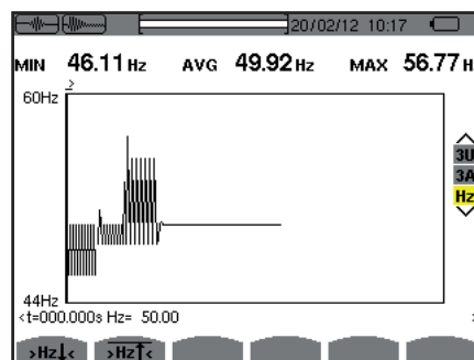
Figura 47: lo schermo di visualizzazione RMS in Hz per un collegamento trifase senza neutro
