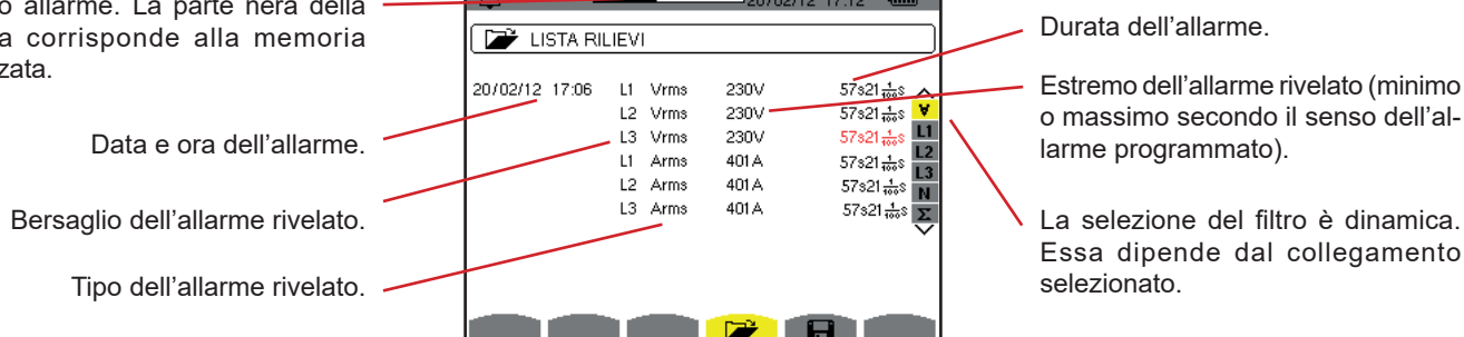
Figura 87: lo schermo Elenco degli allarmi
