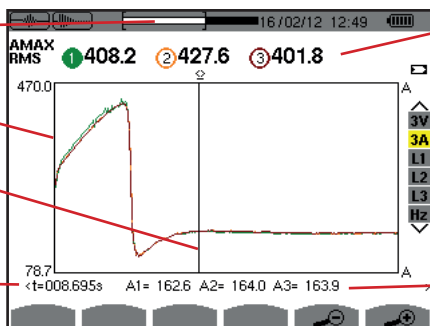
Figura 44: lo schermo di visualizzazione RMS in 3A per un collegamento trifase con neutro
