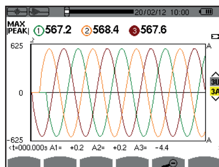
Figura 49: lo schermo di visualizzazione PEAK in 3A per un collegamento trifase a 3 fili
