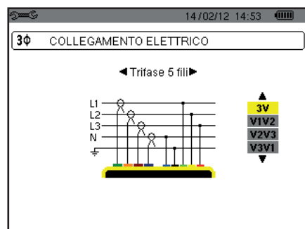
Figura 16: collegamento in trifase a 5 fili
