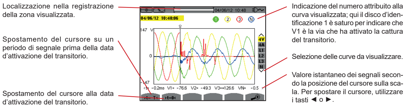
Figura 41: esempio di visualizzazione dei transitori sotto forma di curve in collegamento trifase a 5 fili
