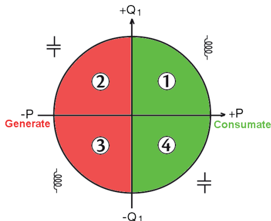
Figura 123: diagramma dei 4 quadranti
