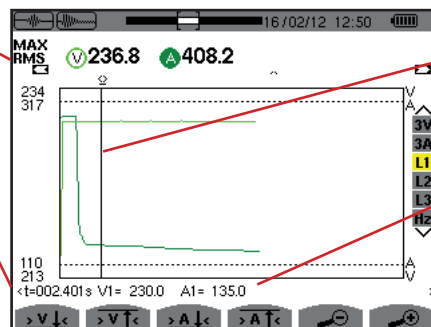
Figura 46: lo schermo di visualizzazione RMS in L1 per un collegamento trifase con neutro
