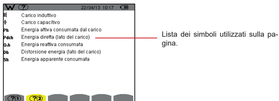
Figura 122: lo schermo di aiuto per il modo potenze ed energie, pagina 2
