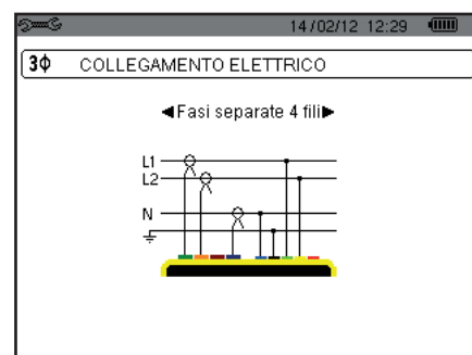
Figura 13: collegamento in bifase a 4 fili
