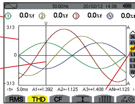
Figura 69: lo schermo di visualizzazione THD in 4A
