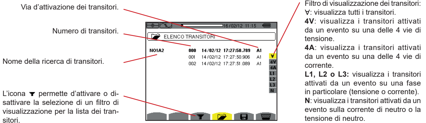
Figura 40: lo schermo Elenco dei transitori in caso di un montaggio trifase a 5 fili
