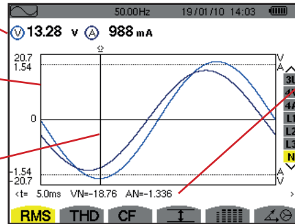
Figura 66: lo schermo di visualizzazione RMS per il neutro
