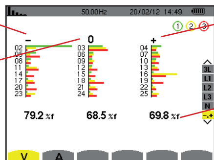
Figura 60: lo schermo del modo esperto per la tensione semplice (montaggi trifasi con neutro)
